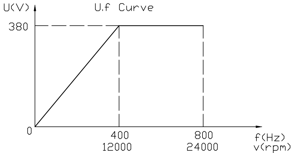
频压曲线
